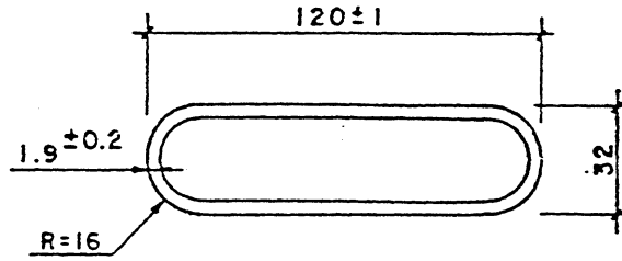
SECCION B-B
