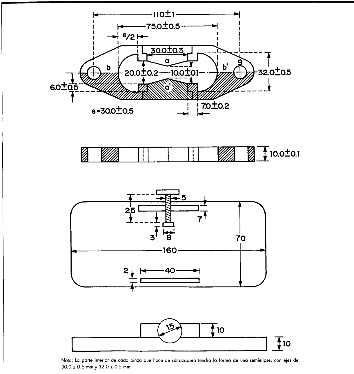
Figura 1.-Molde y placa para Ductilómetro. Medidas en mm.
