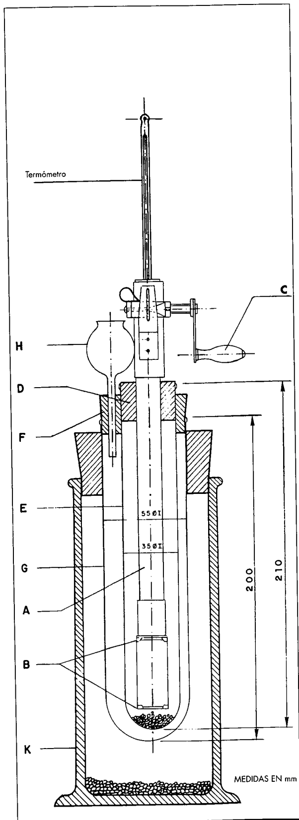
Figura 1.-Conjunto del aparato.
